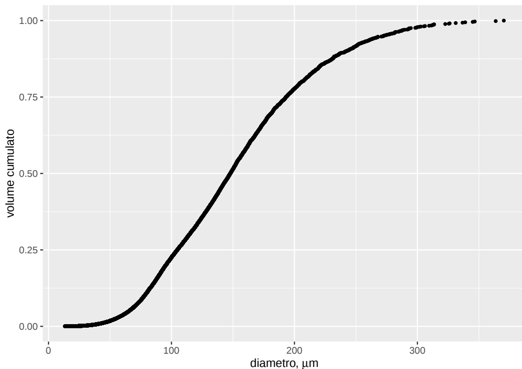
Figura 4.1: Curva del volume cumulato delle gocce.
