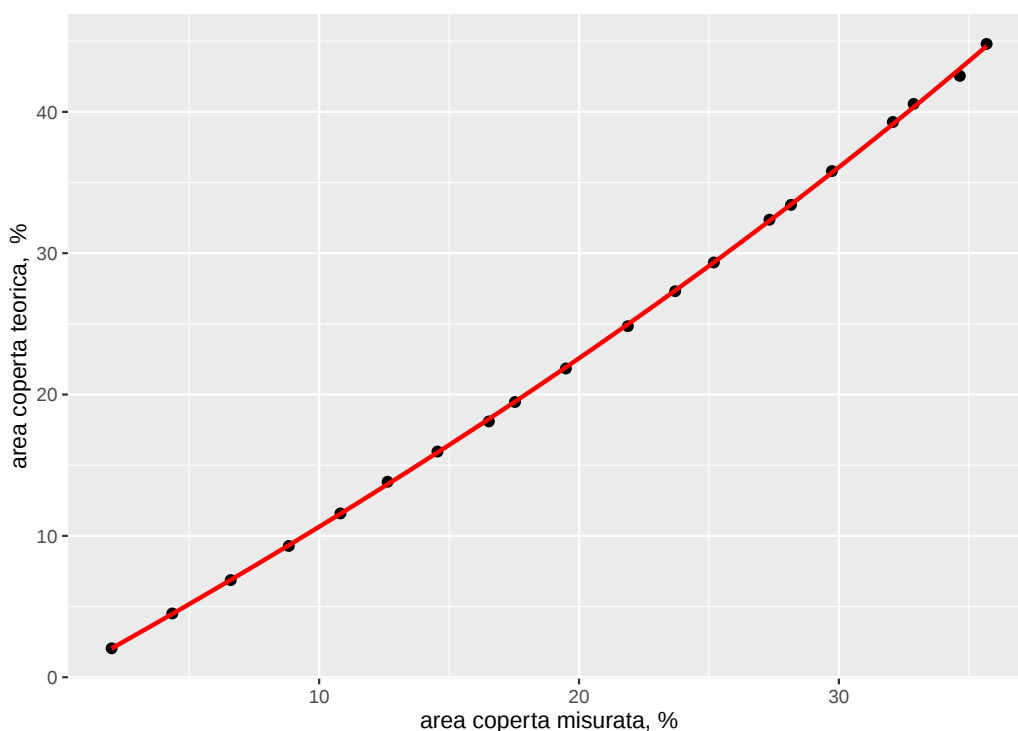
Figura 4.3: Relazione fra area coperta teorica e area coperta misurata.
