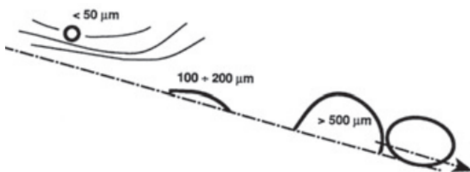
Figura 2.2: Comportamento delle gocce sulla superficie fogliare in funzione delle dimensioni.
